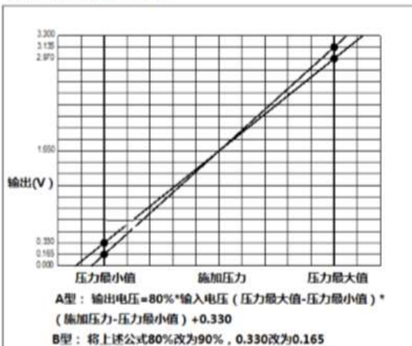
压力转换方程, 电压输入3.3V
