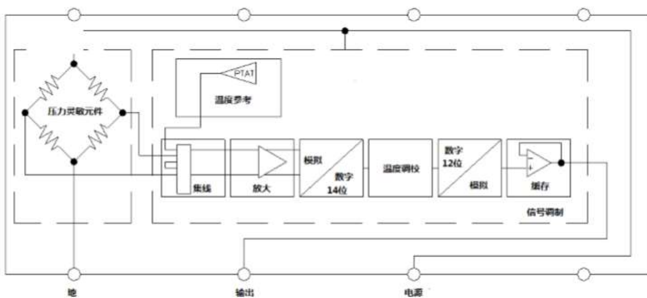
LW19 模拟放大输出等效电路
