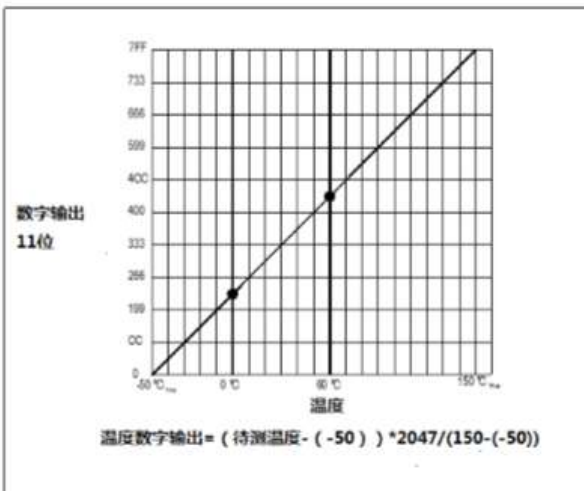
温度转换方程
