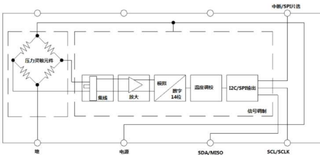
LW19 数字输出等效电路
