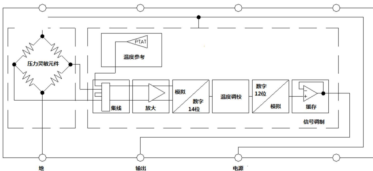
LW52 模拟放大输出等效电路
